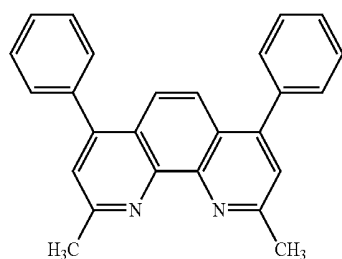
BCP
